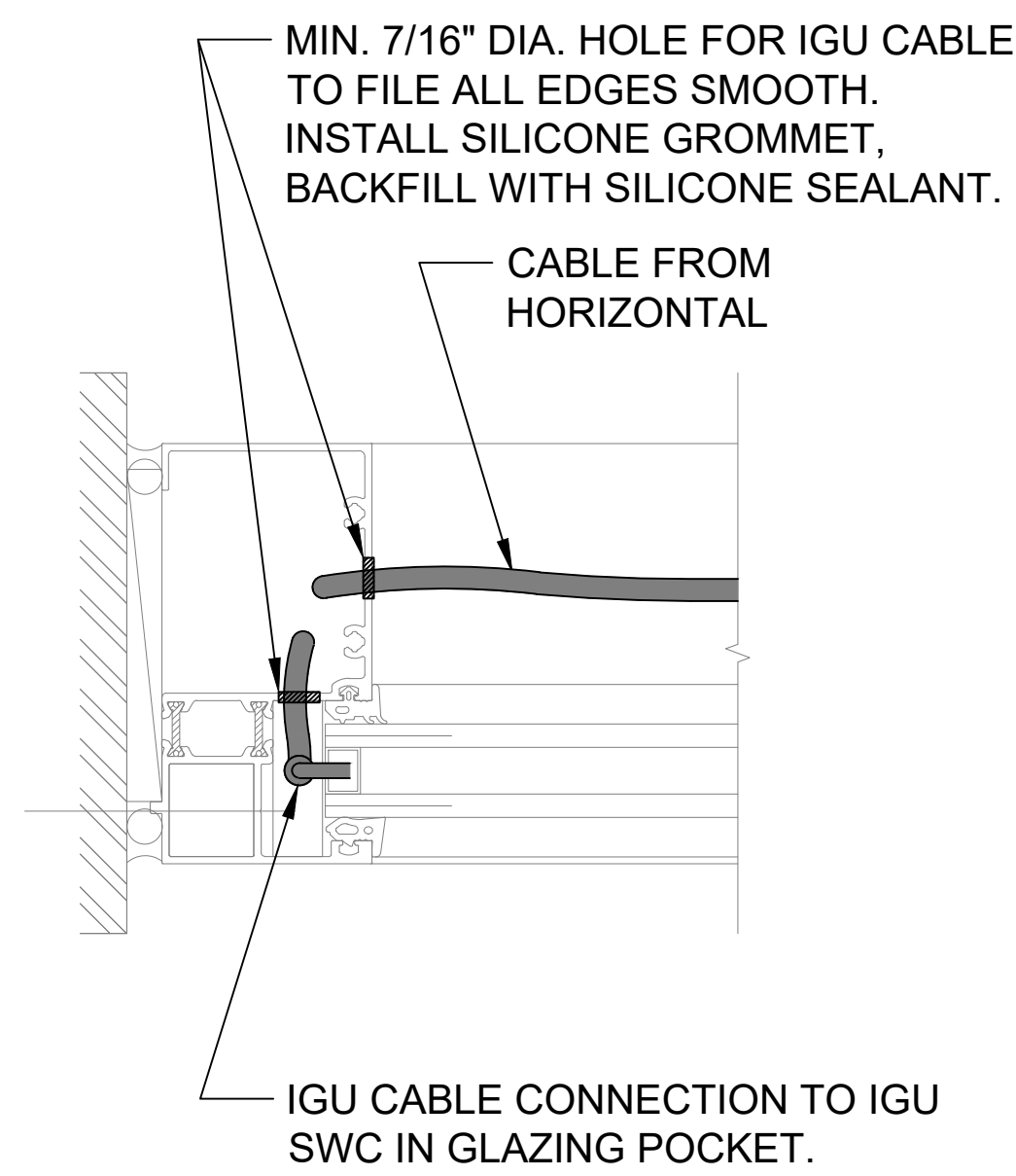
DETAIL 4 LEFT JAMB
